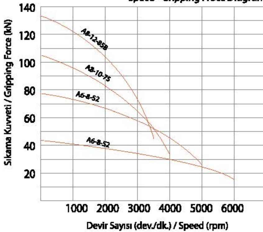
Devir Sayısı - Sıkma Kuvveti Speed - Gripping Force Diagram
